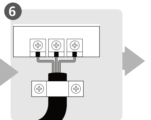
Kablo Bağlama
